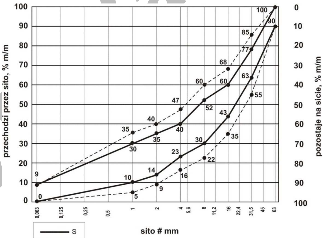
Rys. 4. Mieszanka niezwiązana 0/63 mm do warstw podbudowy zasadniczej nawierzchni obciążonej ruchem kategorii Ko3,2 (poniżej KR3)
